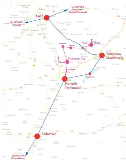
Rysunek 3. Schemat lokalizacji punktów styku sieci Internetowej w konsorcjum gmin E-leader.
